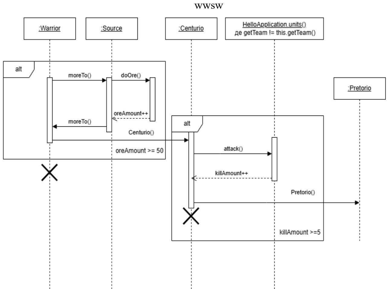
Рисунок 3.6 – Діаграма послідовності
