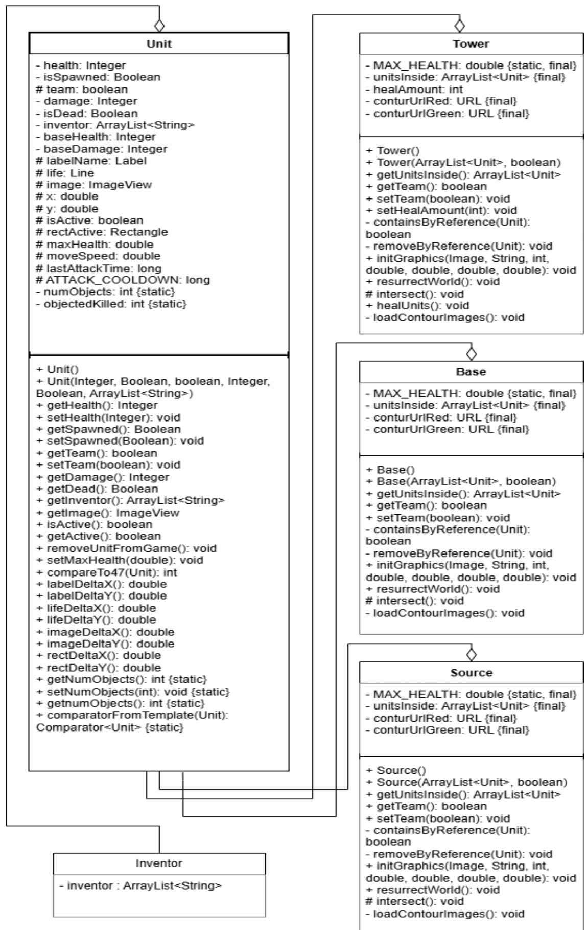
Рисунок 3.1 – Діаграма наслідування
