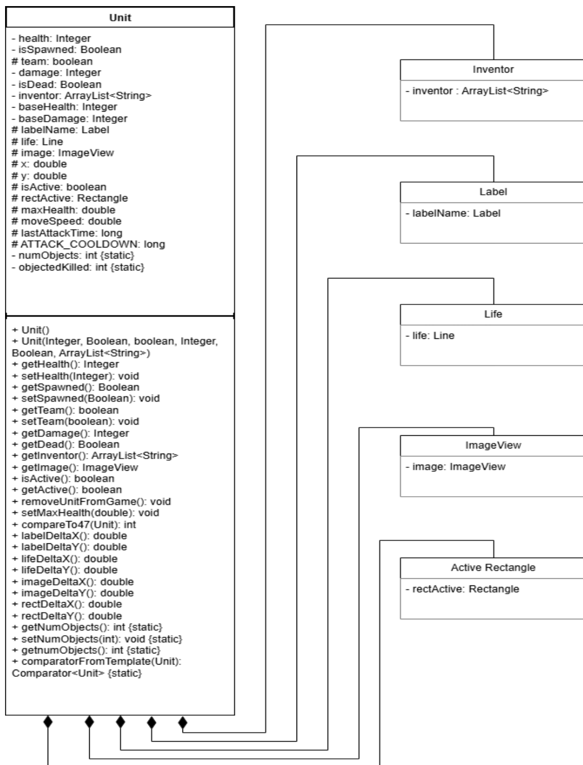
Рисунок 3.3 – Діаграма композиції
