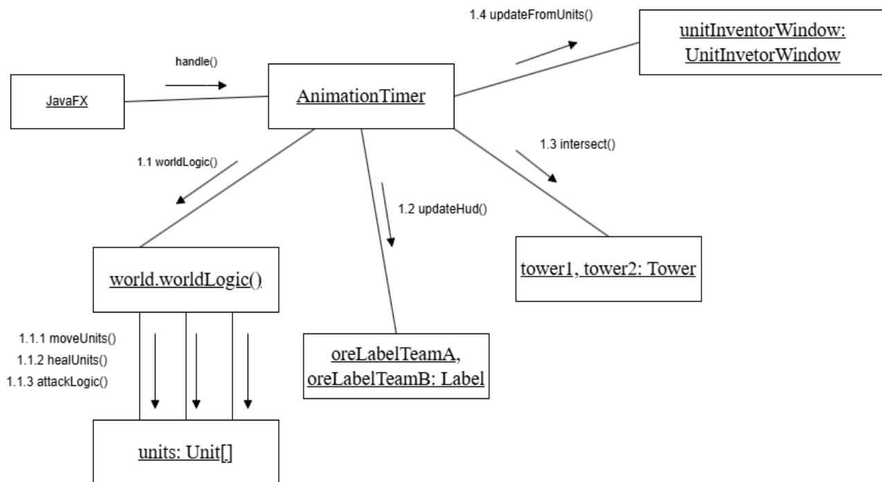
Рисунок 3.5 – Діаграма кооперації
